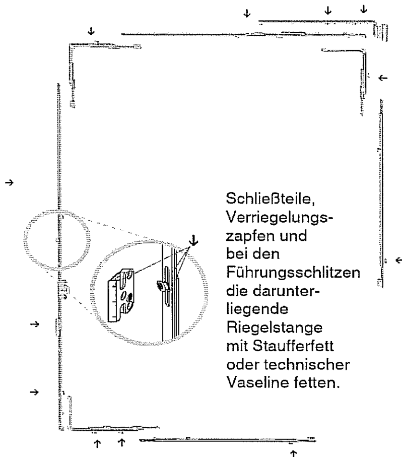
Beispiel Dreh-Kipp-Beschlag (DK)
