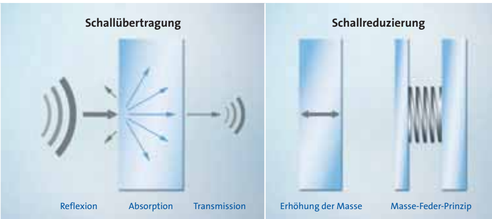
Mit zunehmender Dicke des Glases und Asymmetrie erreicht man hohe Schalldämmwerte. Zwei Scheiben, die als Masse-Feder-Prinzip zu einem Isolierglas verbunden sind, addieren sich in den Frequenzverläufen zu einer besseren Schalldämmung.
